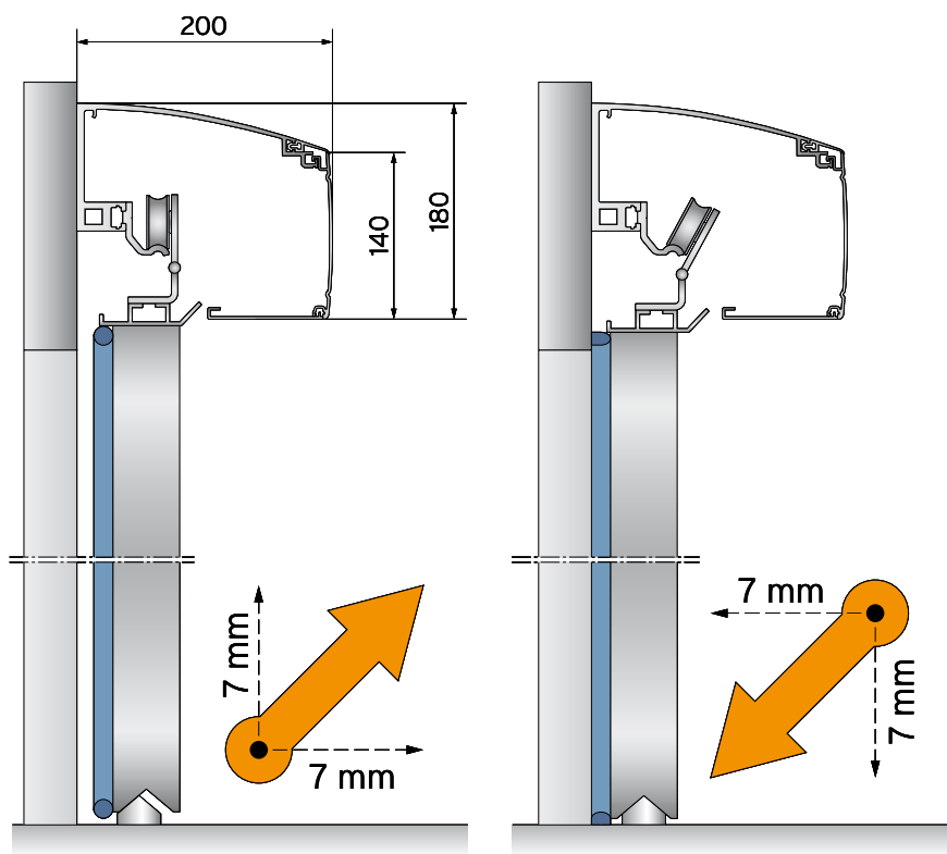
Automatismo SLX-D con cobertor de limpieza fácil, carro de rodamiento ajustado para la operación normal.
